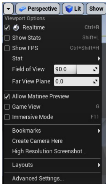
Bild 3.7 Die Viewport-Optionen
