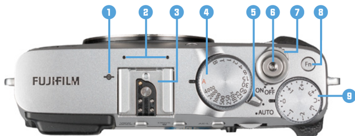
▲ Bedienelemente auf der Oberseite der X-E3.
