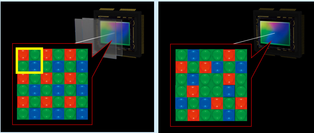
▲ Links: Farbfilter nach dem Bayer-Schema mit vorgelagertem Tiefpassfilter. Rechts: FUJIFILM X-Trans™-Architektur ohne Tiefpassfilter (beide Bilder: FUJIFILM).
